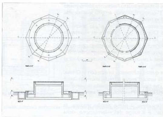
PIANTE E SEZIONI DELLA VASCA A TRACIMAZIONE
