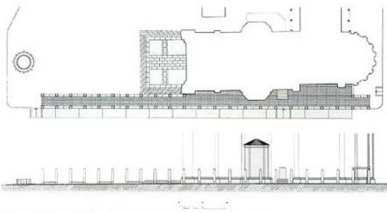
PIANTA E PROSPETTO DEL COLONNATO E DELLA VASCA A TRACIMAZIONE REALIZZATI PRESSO LA CHIESA
